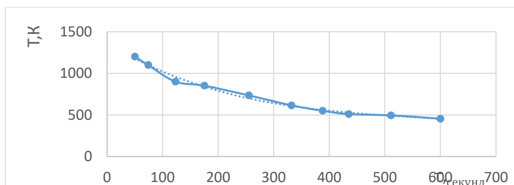
Рис.1. Зависимость изменения температуры образцов (Т) от времени охлаждения (τ) для медного образца (7,517гр), [11].
