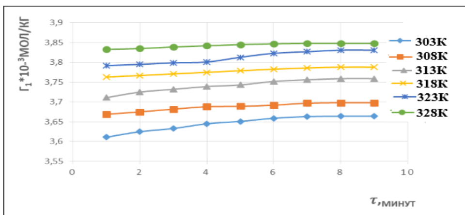
Рисунок 1. Зависимость изменения адсорбции исследуемых объекта (1гр флюорита) от температуры и времени
