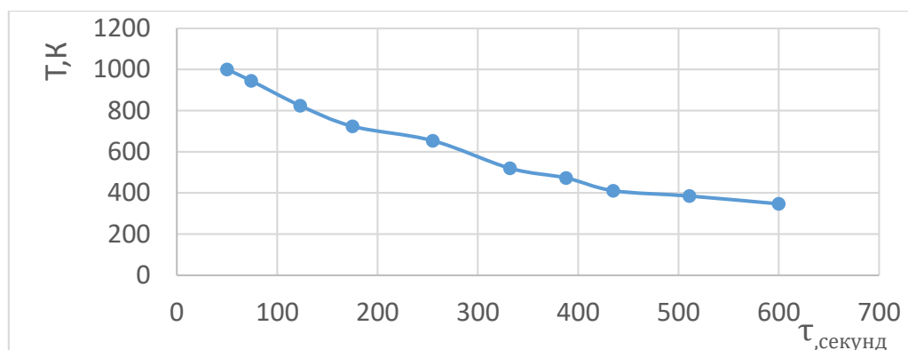
Рис.2. Зависимость изменения температуры образцов ( T ) от времени охлаждения ( \tau ) для флюорита марки ФК-70 (0,918гр), [11].
