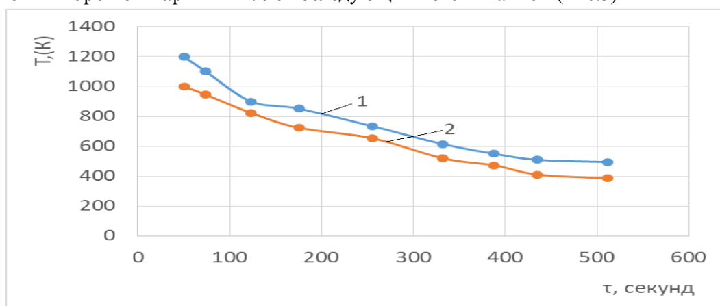
Рис 3. Зависимость изменения температуры образцов (Т) от времени охлаждения (τ) ((эталон мед —1) и наш образец — 2) [5, 8, 10].
